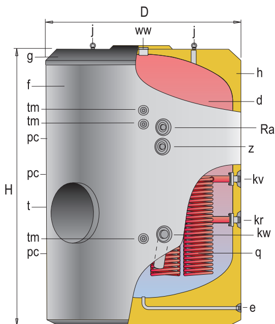
Modelo de 6000 litros con patas
